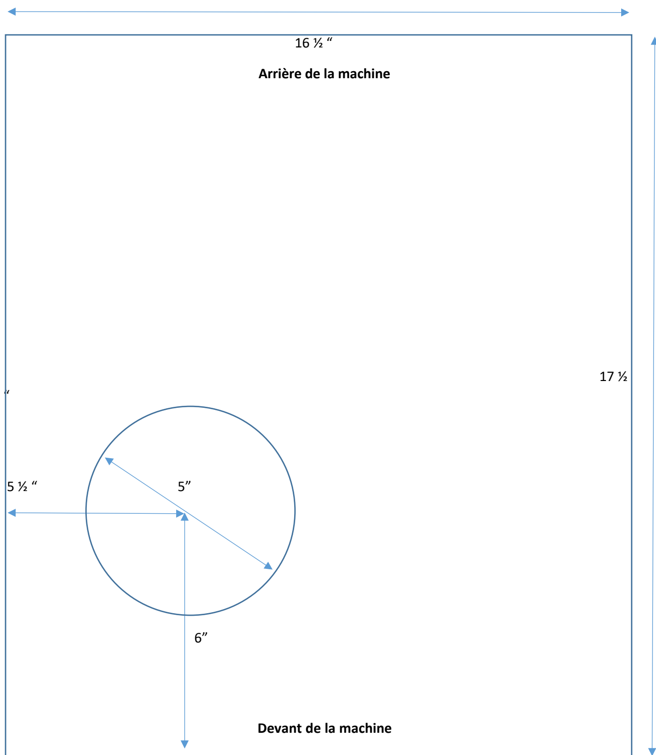
Gabarit de perçage du trou de chute à déchet - Wittenborg 9100
