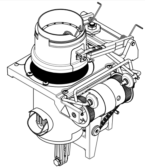
06CAB22 PLATINUM BREWER ASSY ASSEMBLAGE INFUSEUR PLATINUM
