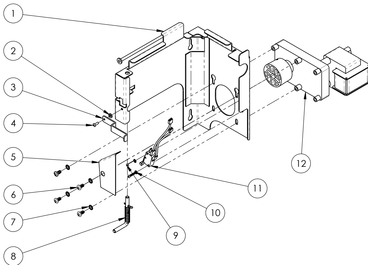
PEASS20 BREWER BRACKET S-A S-A SUPPORT INFUSEUR
